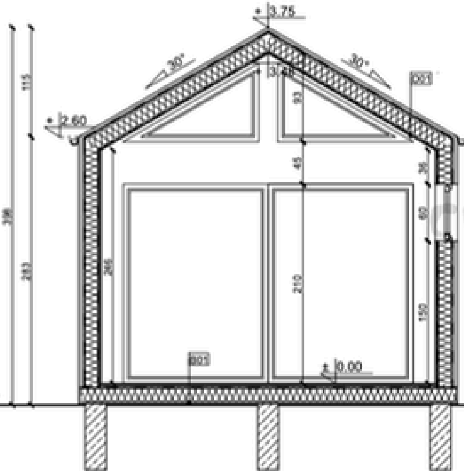
PRZEKRÓJ 1-1 / SCHNITT 1-1
