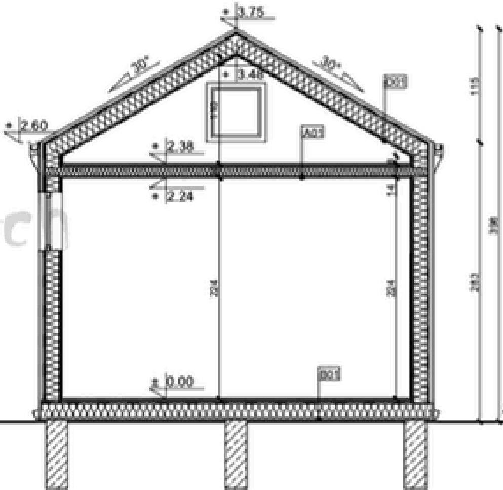
PRZEKRÓJ 2-2 / SCHNITT 2-2
